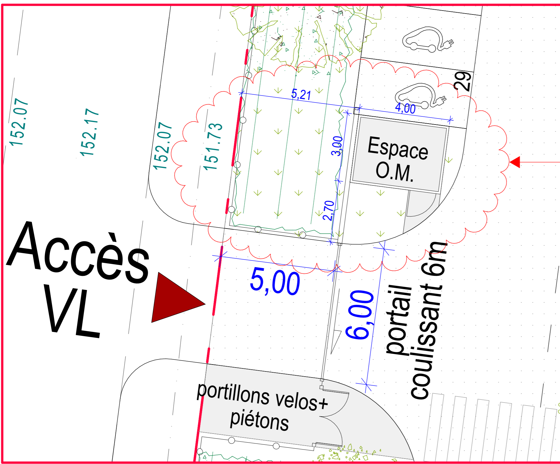
agrandissement sur l'espace ordures ménagères (O.M.) 1:100°
